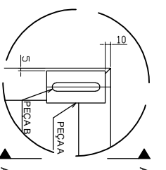
DETALHE A OLHAL DE SUSTENTAÇÃO
